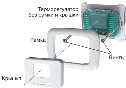
Рис. 10 Установка терморегулятора
